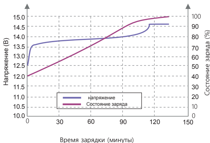
Кривая состояния заряда (0,5 ° С, 25 ° С)
