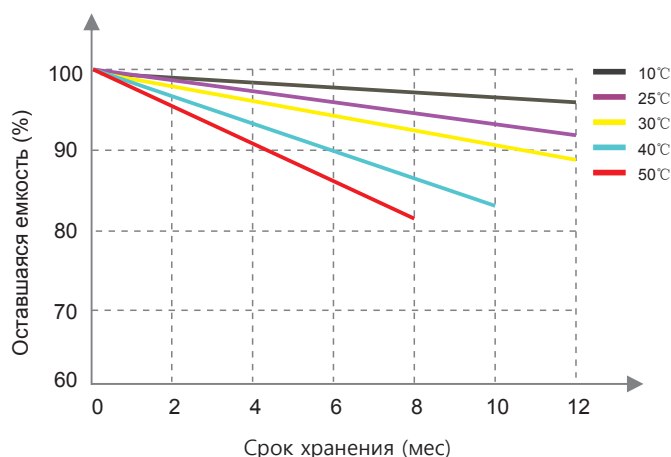
Кривая саморазряда при различных температурах
