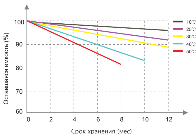
Кривая саморазряда при различных температурах
