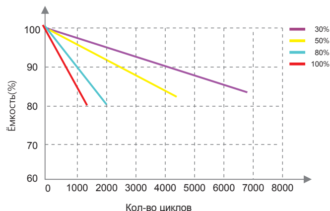
Влияние глубины разряда на срок службы
