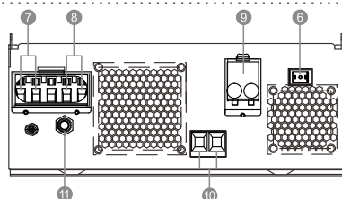
2-5.5кВт одиночна модель
