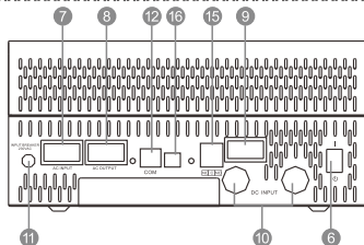
3-5.5кВт одиночна модель
