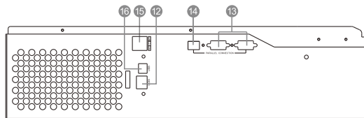
2-5.5кВт паралельна модель
